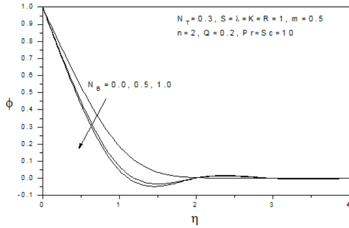
Fig.2 (d) Concentration profiles for different values of N_B
