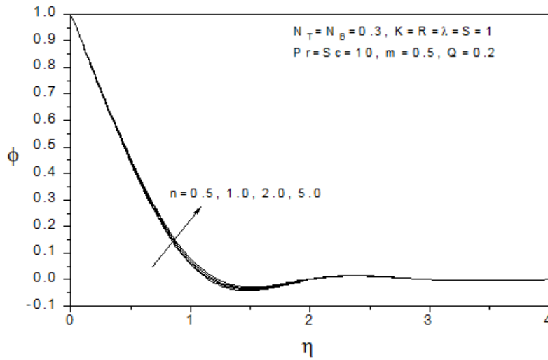
Fig.3 (d) Concentration profiles for different values of n
